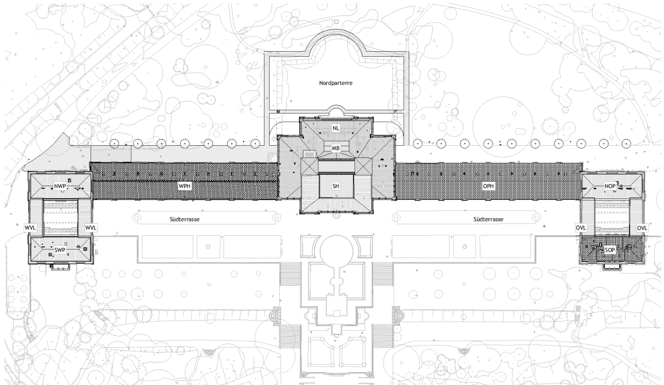
Abb. 01 SN_OR110G-03_A300_LA003-2.pdf Lageplan Orangerie Bestand
