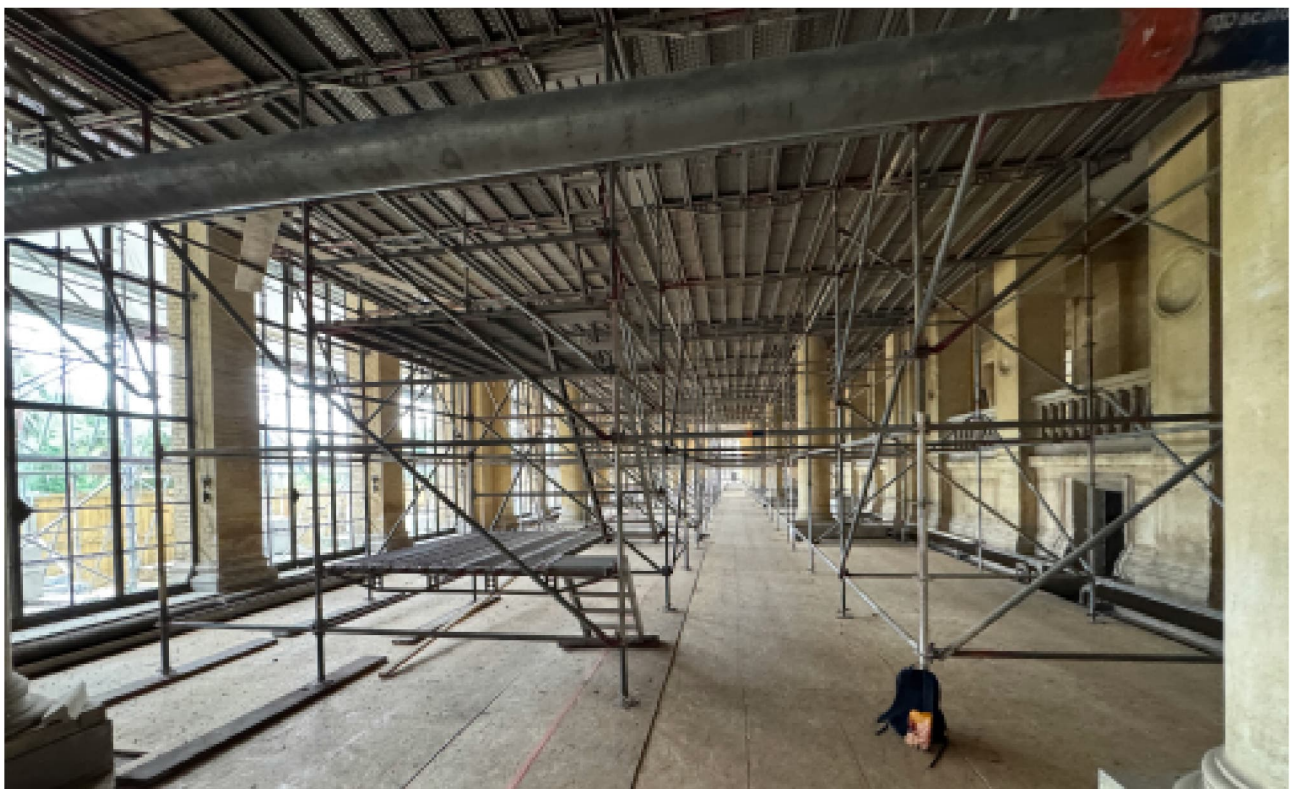
Abb. 28 2025-07-08 ML_008 OR.JPG Östliche Pflanzenhalle - Raumgerüst, Teilaufbau noch ohne Arbeitsebenen, nach Baubeginn Sanierung Dachstuhl 2025
